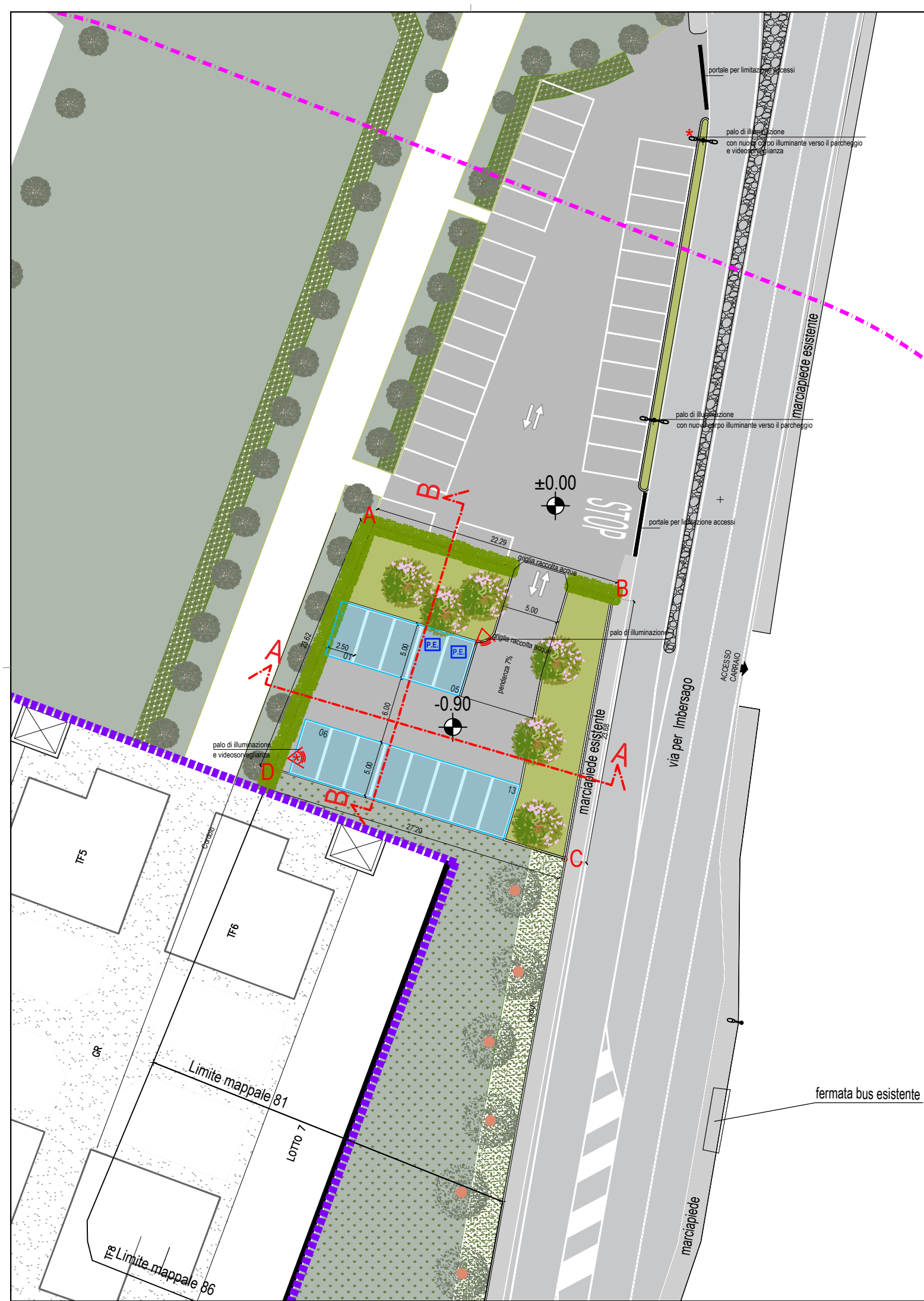
PLANIMETRIA
