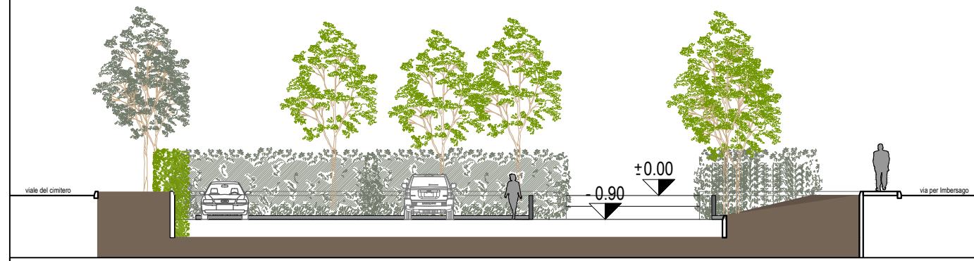
SEZIONE A-A
